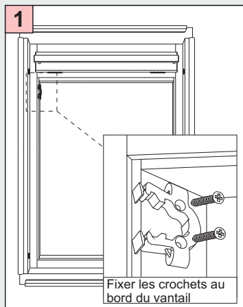
Réglage Supports de Fixation
