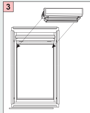
Montage de la Cassette
