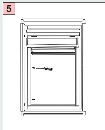
Fixation des Guides latéraux
